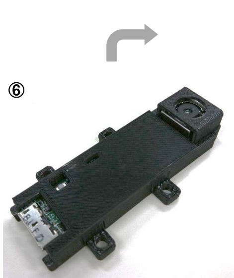
6. Overlay the top lid.
