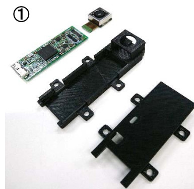
① 各パーツ
