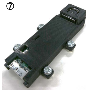
⑦ M3のネジとナットを組込んで完成。
