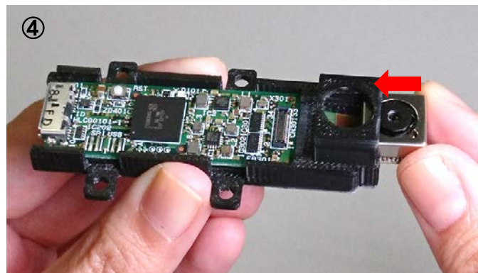
④ カメラのヘッド部を持ち、水平に挿入。 ！基板とカメラのコネクタがぶつからないように注意。
