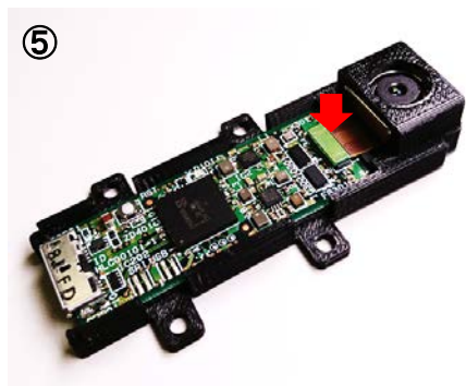
⑤ 基板とカメラのコネクタを結合。 ！コネクタを強い力で無理に押さえ込まない。
