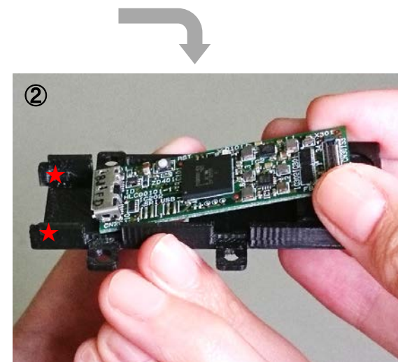
② 基板を斜めの角度で★部のスリットに差し込む。
