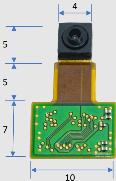
(単位：mm) ヘッド部：H 3.5 チップ部：H 1.1
